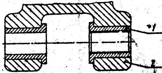
1 - втулка; 2 - корпус
